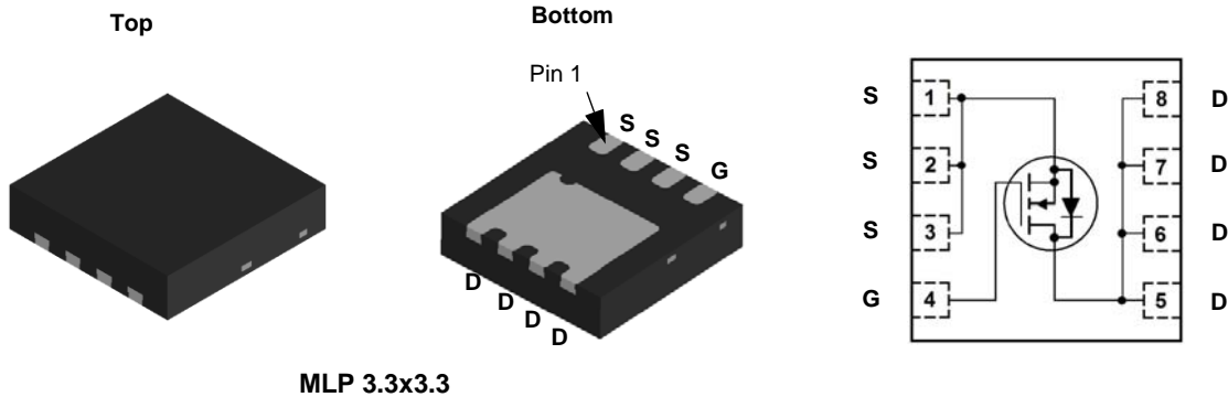
MLP 3.3x3.3
