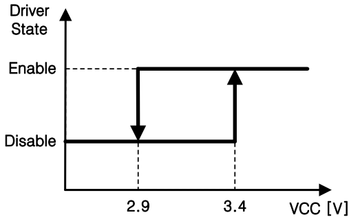
Figure 28. UVLO
