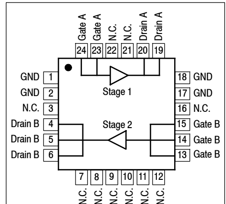
QFN 4 × 4
