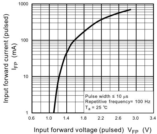
Fig. 11.6 I_{FP} - V_{FP}
